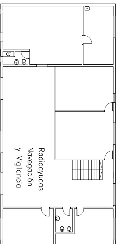
PLANTA ALTA
