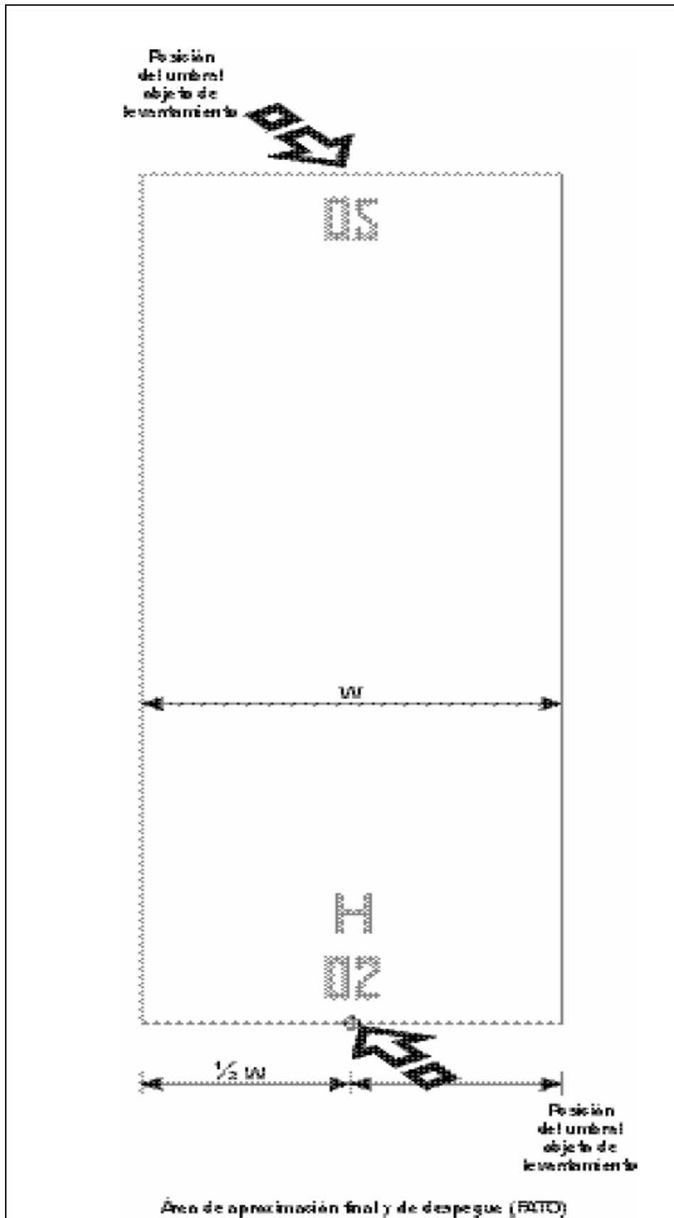
B.5 Posición de la FATO de umbral en el plano objeto de levantamiento geodésico
