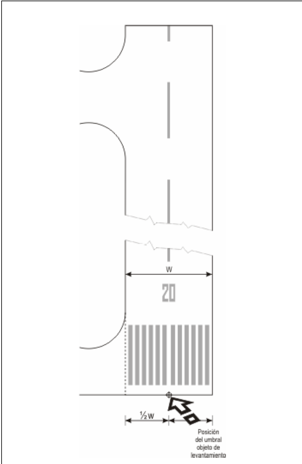
B.3 Posición del umbral en el plano objeto de levantamiento geodésico
