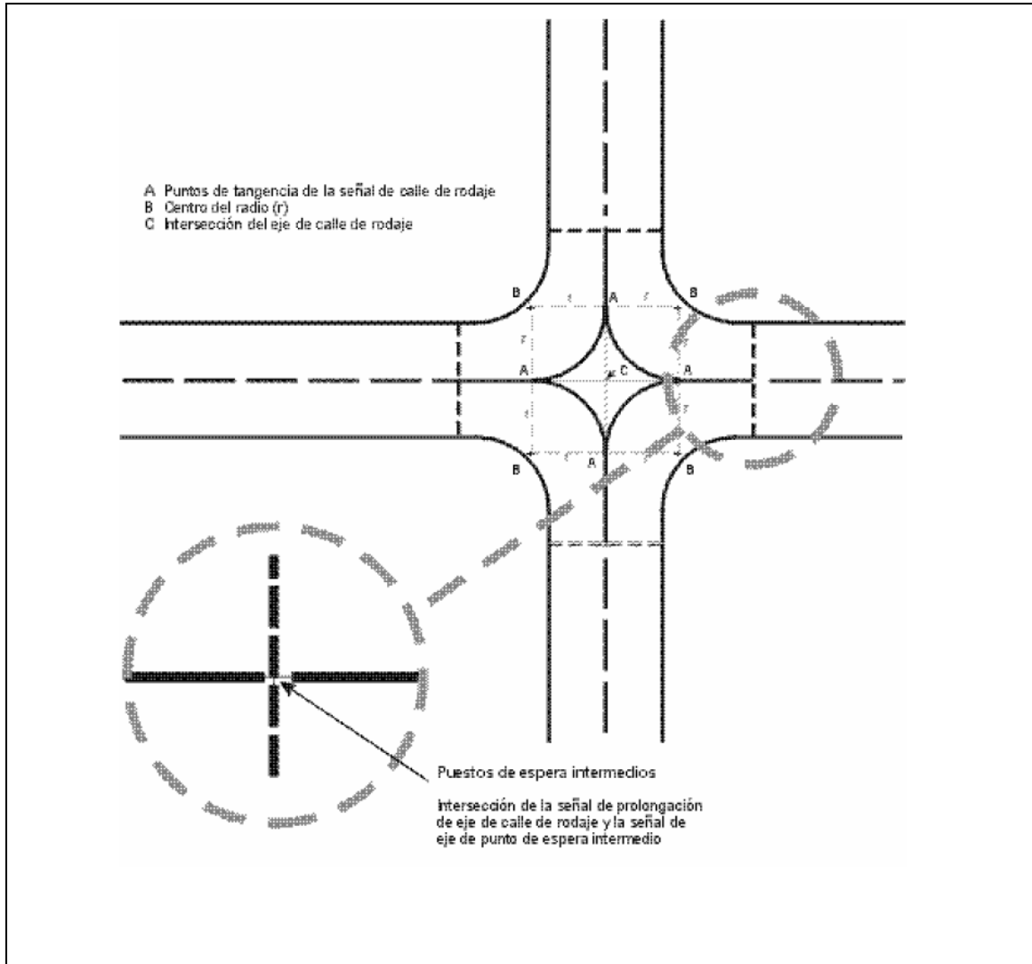
B.9 Intersecciones de calle de rodaje
