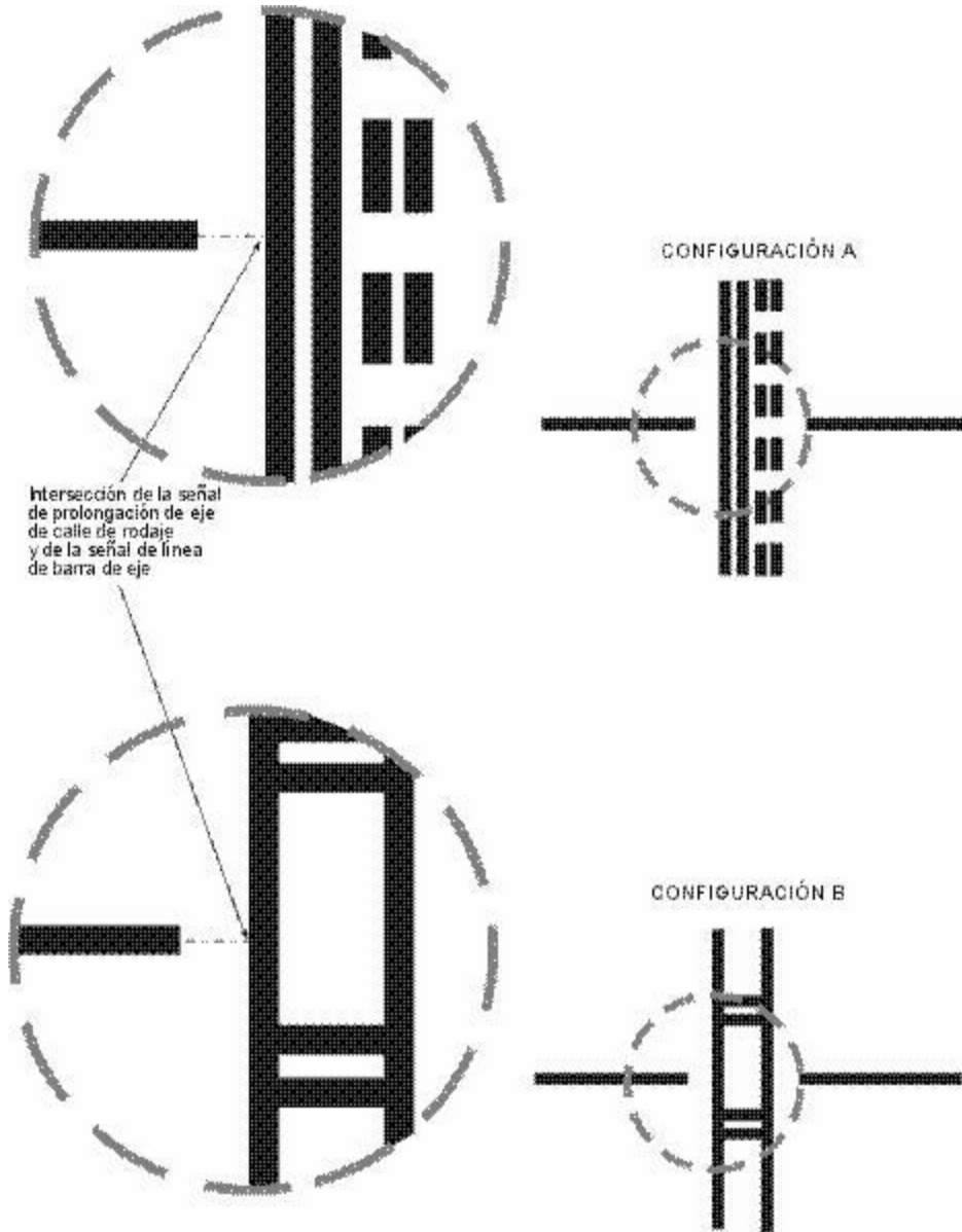
B.8 Puntos de espera
