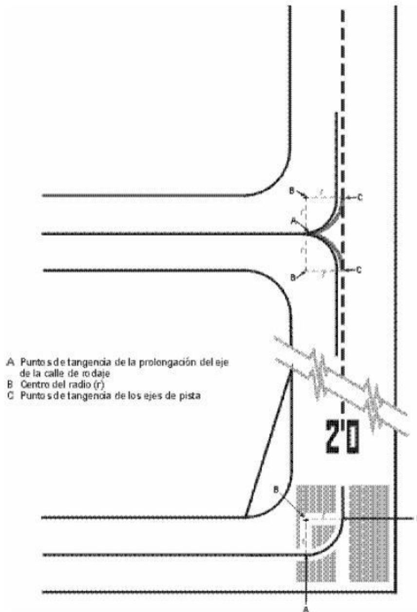
B.6 Intersecciones de pista y calle de rodaje
