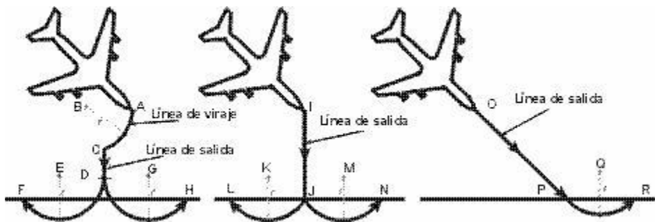
B.13 Líneas de proa de entrada desplazada
