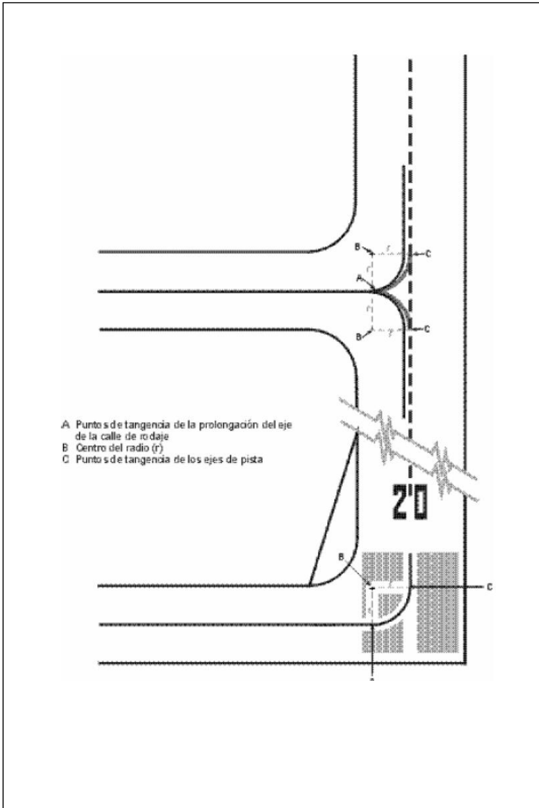
B.7 Intersecciones de pista y calle de rodaje
