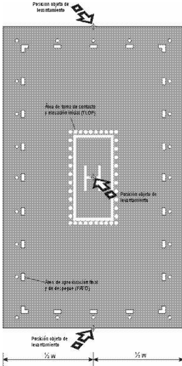
B.4 Posiciones de las TLOF y FATO de umbral en el plano objeto de levantamiento geodésico
