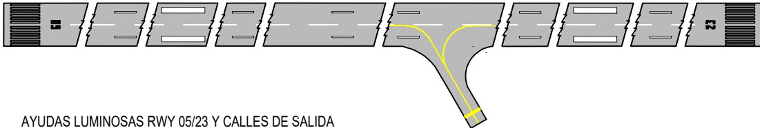
AYUDAS LUMINOSAS RWY 05/23 Y CALLES DE SALIDA
