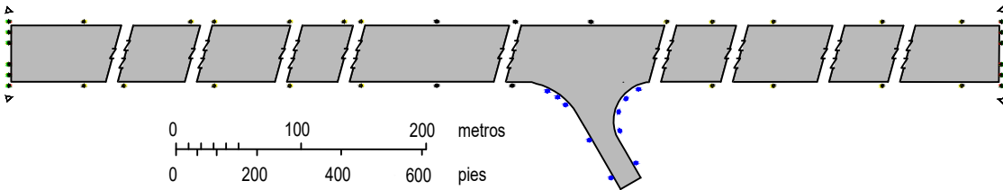
AYUDAS LUMINOSAS RWY 05/23 Y CALLES DE SALIDA
